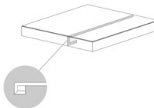
ANGULO GRADONE RECTO 20MM SP2099 | 60X60 / 24"x24"
